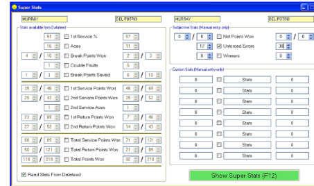
SuperStats Interface
